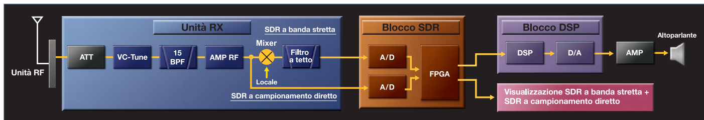
Configurazione SDR ibrida
