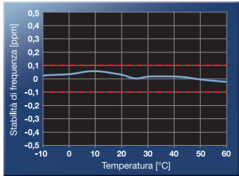
Stabilità in funzione della temperatura del TCXO
