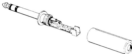
AUTO KEY (Paddle) Plug
