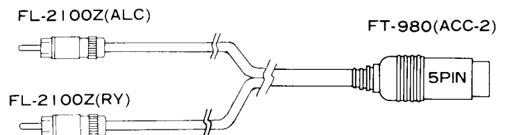
OPTIONAL CABLE
