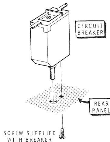
Detail 13-8E
