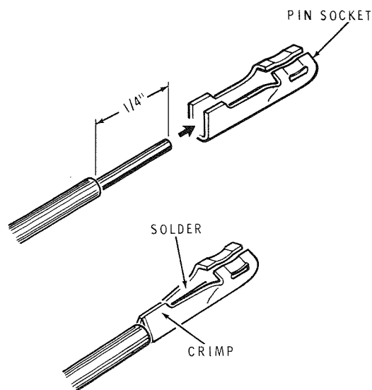
Detail 13-15E
