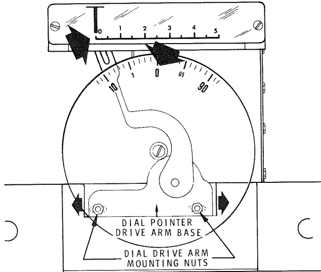
Detail 13-16E
