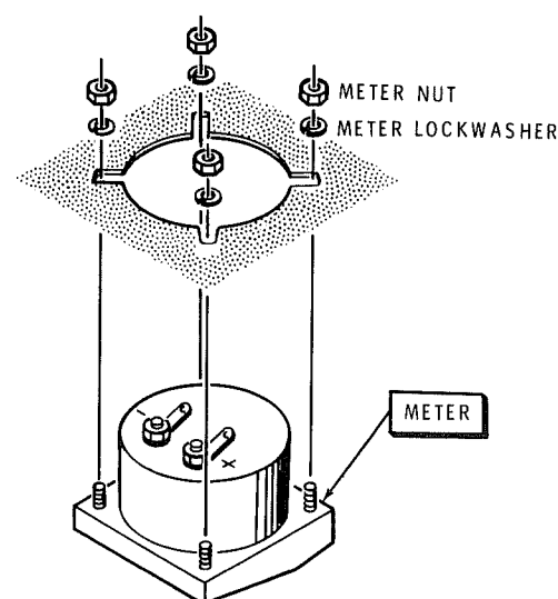
Detail 13-17E
