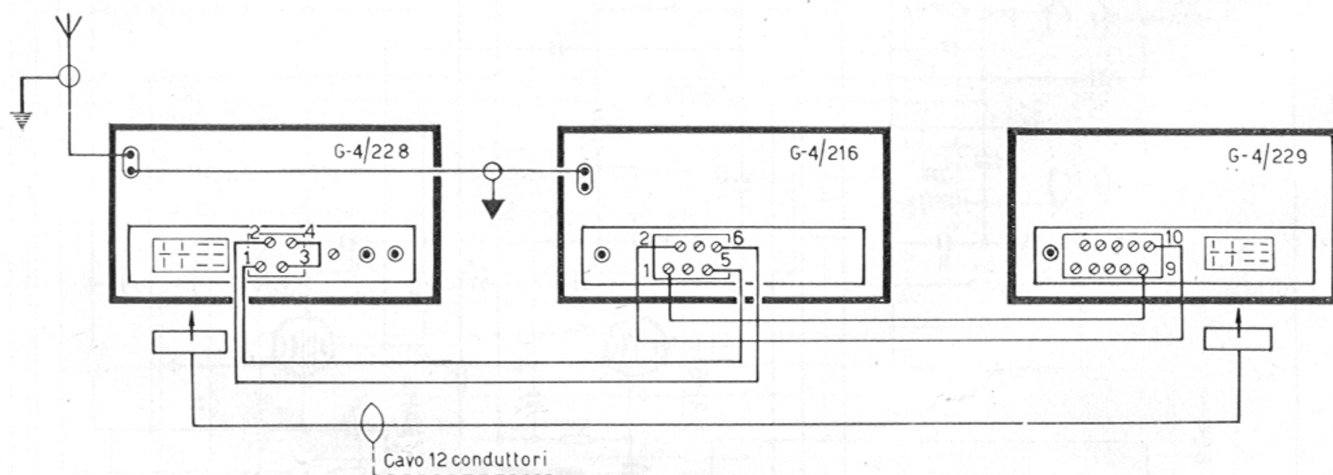
Schema di collegamento per funzionamento manuale
