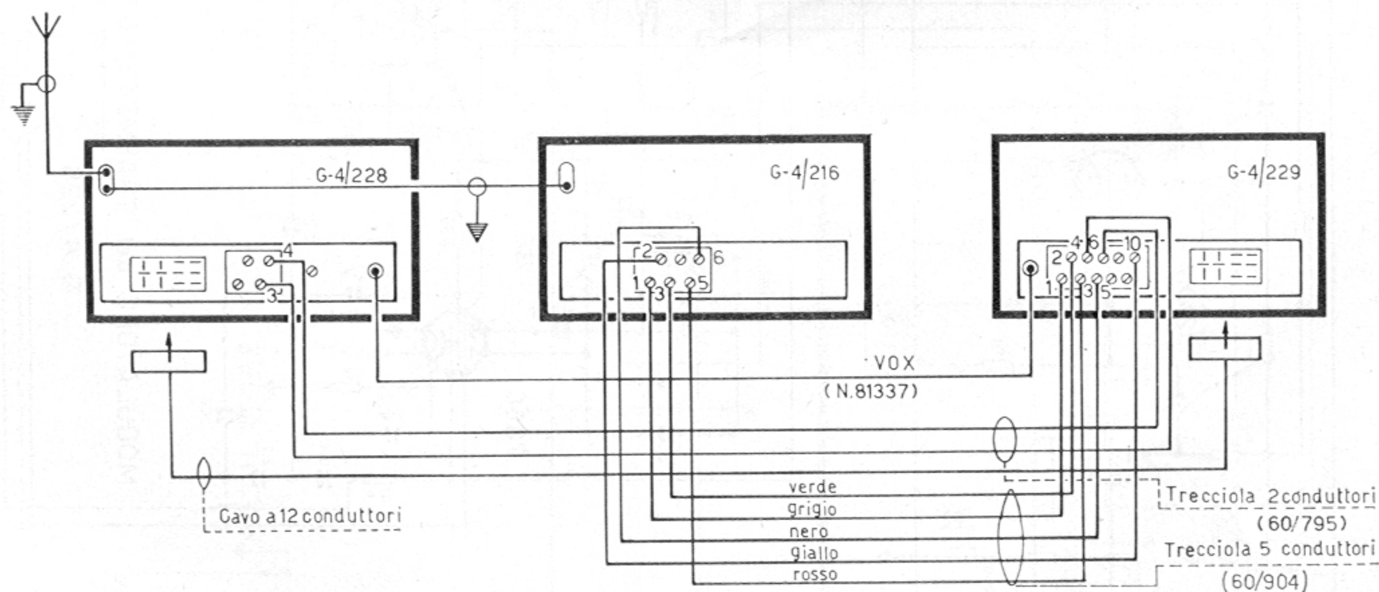
Schema di collegamento per funzionamento automatico
