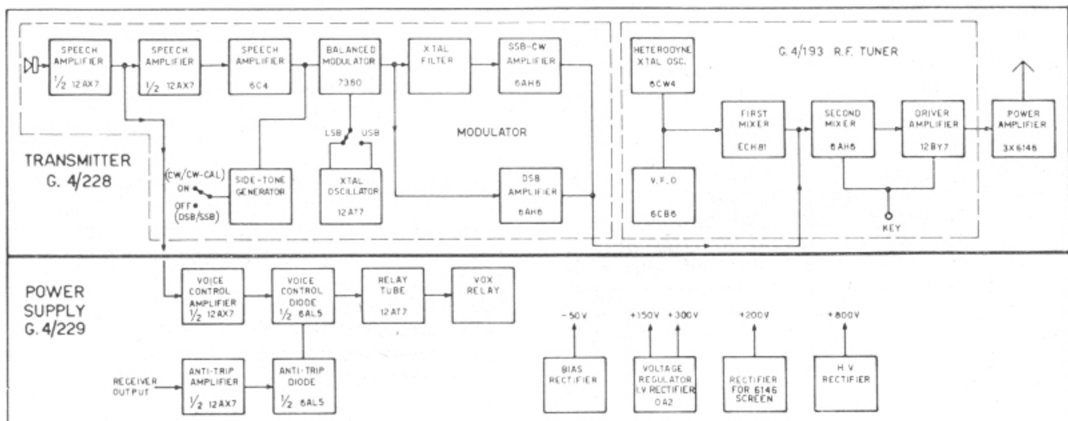
Schema « a blocchi » del trasmettitore.
