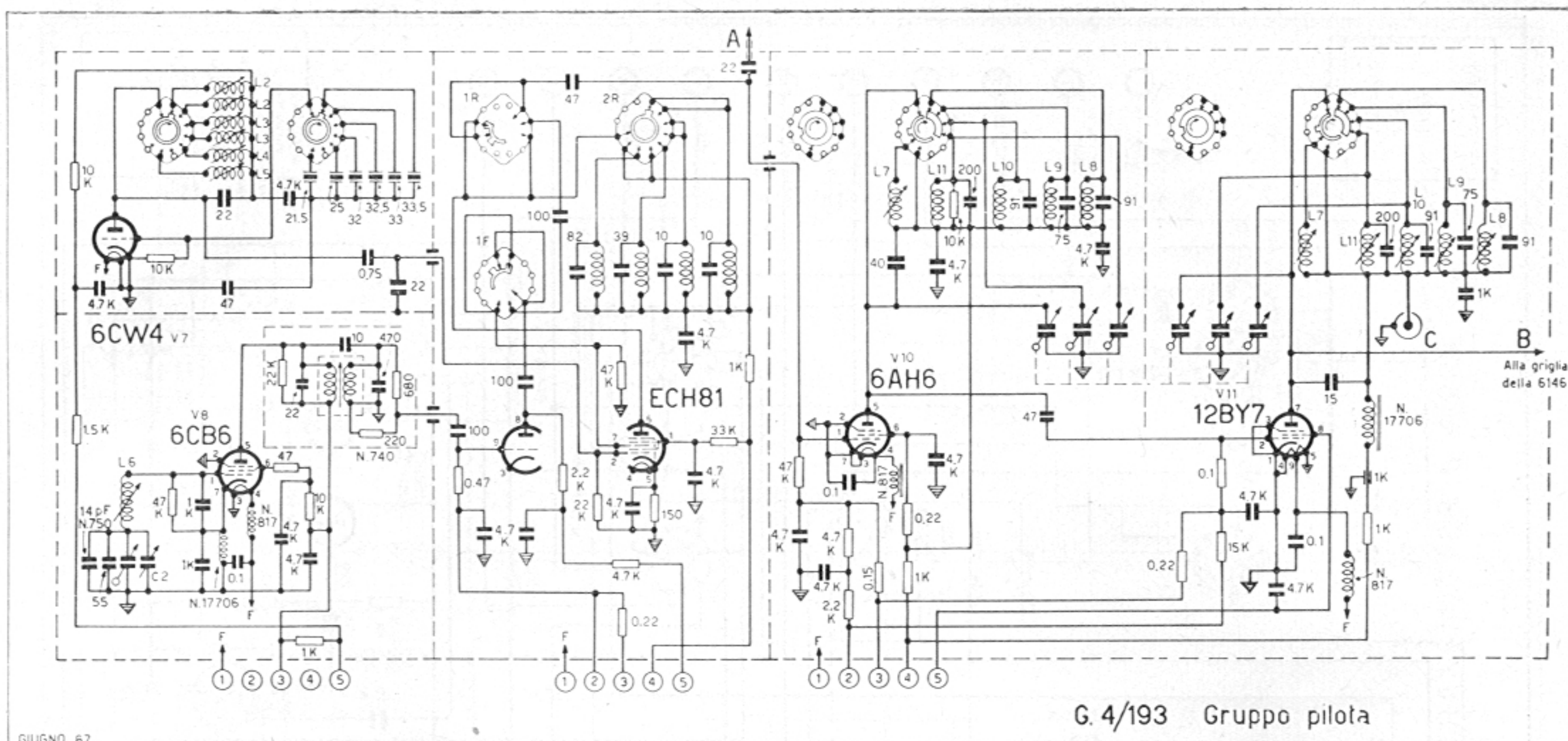
Schema elettrico gruppo pilota 4/193
