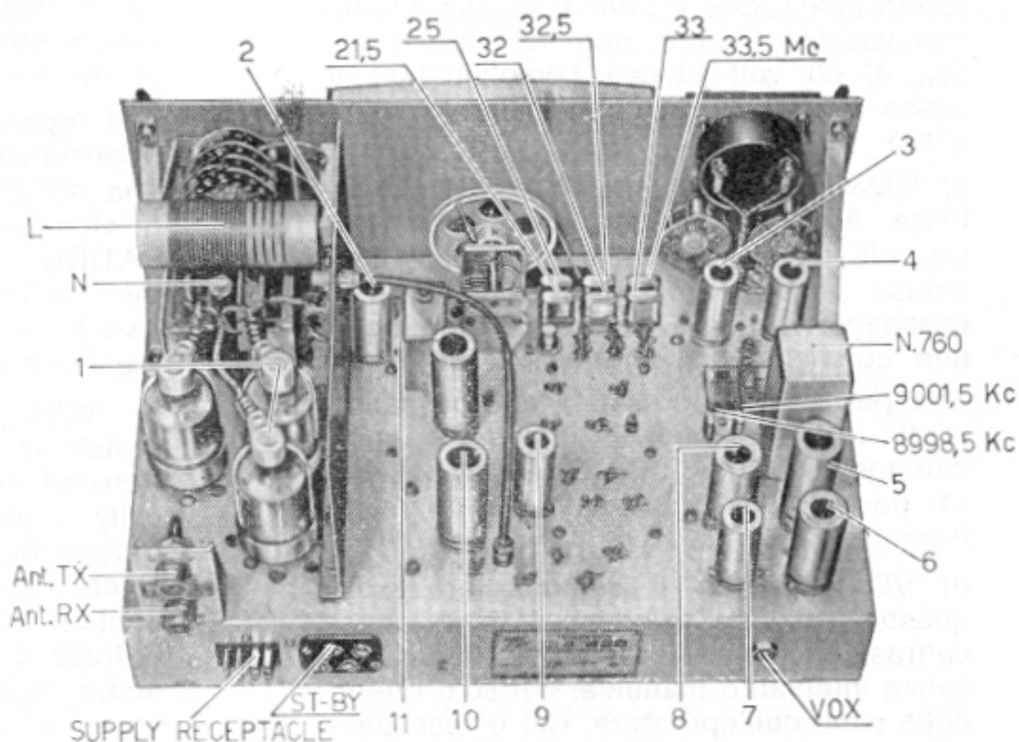
Vista posteriore del trasmettitore G 4/228
