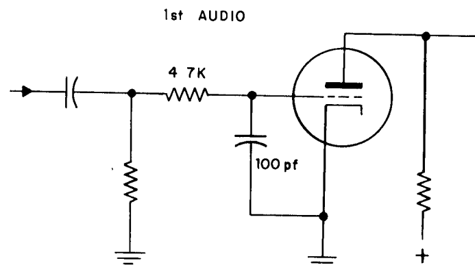
R-C R.F. FILTER
