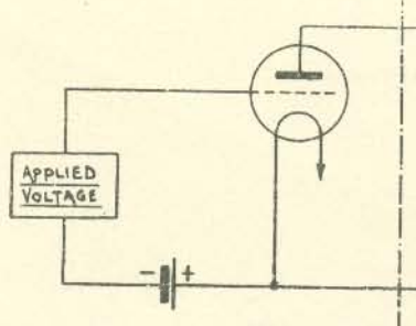
FIG. 18. Battery bias.
