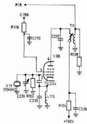
Sl. 22 — Kristal-oscilator 17,5 MHz
