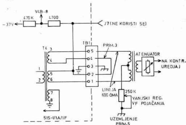
B. SPOJ SA LINIJOM OD 600 OMA I UZEMLJENOM SREDNJOJ TAČKOM TRANSFORMATORA
