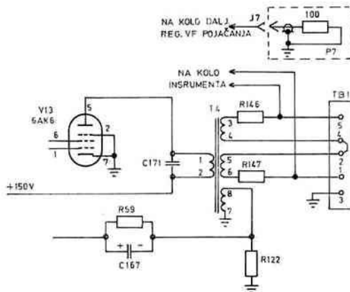
Sl. 8 — Šema veza izlaznog stepena prijemnika 51S-1B
