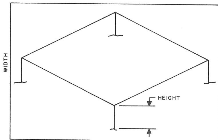
LENGTH RHOMBIC
