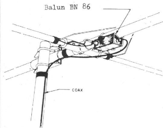
Fig. 7. - Fixation du balon.
