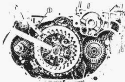
1. Clutch holding tool 1. Outil de maintien d'embrayage 1. Kupplungs-Haltewerkzeug
