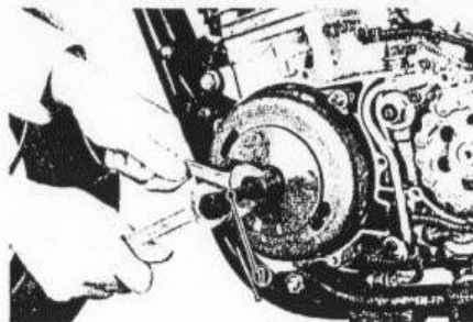
1. Flywheel puller 2. Extracteur de volant 1. Schwungrad-Abziehwerkzeug
