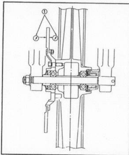
1. Dial gauge 1. Comparateur à cadran 1. Meßuhr
