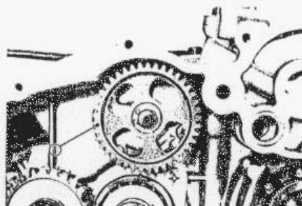
1. Pump driven gear 1. Pignon mené de la pompe 1. Pumpenantriebsrad
