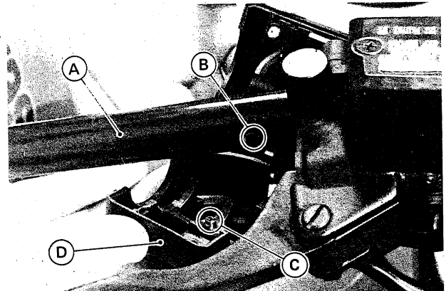
A. Lenker
