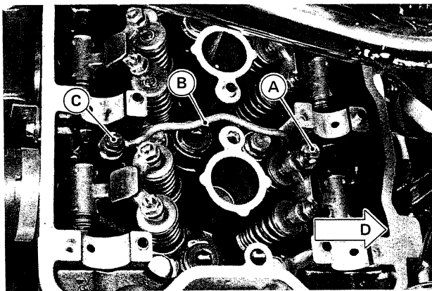
A. Weiße Schraube B. Zylinderkopf-Ölleitung C. Schwarze Schraube D. Auslaßseite
