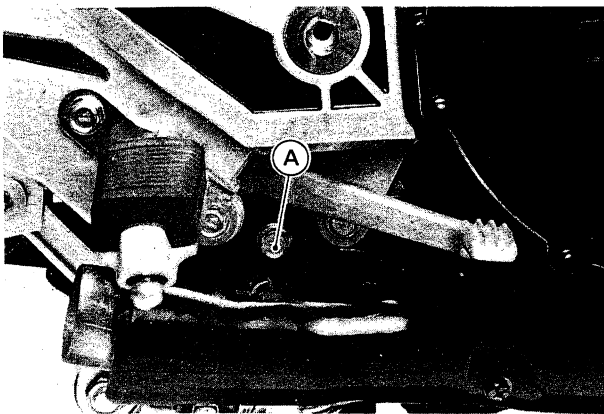
A. Auspuffrohr-Befestigungsschrauben
