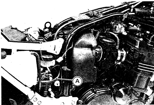
A. Reservetankschlauch
