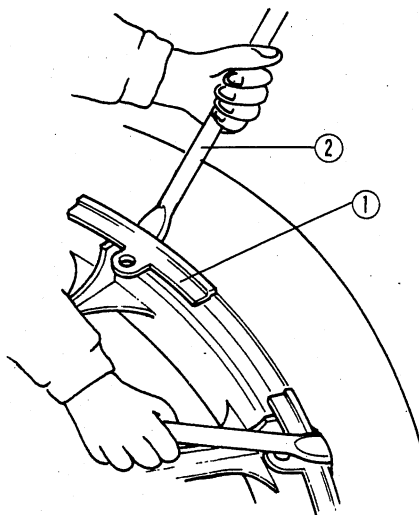
1. Reifenschoner: 57001-1063 2. Montiereisen: 57001-1073
