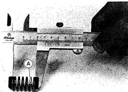
A. Kupplungsfeder
