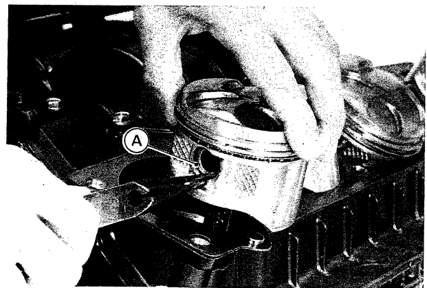
A. Sicherungsring
