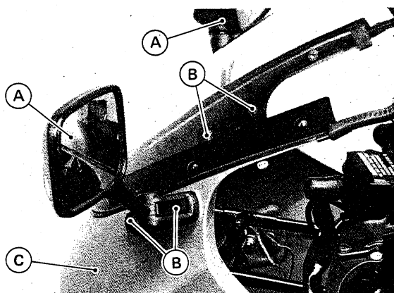
A. Rückspiegel B. Befestigungsschrauben C. Obere Verkleidung
