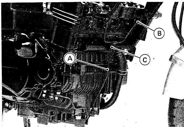
A. Hauptölleitung B. Hohlschraube C. Befestigungsschraube
