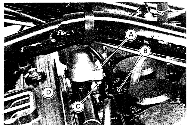
A. Choke-Zug B. Klemmschraube
