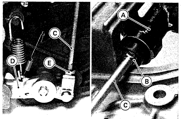
A. Hauptzylinder
