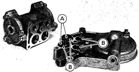
B. O-Ringe
