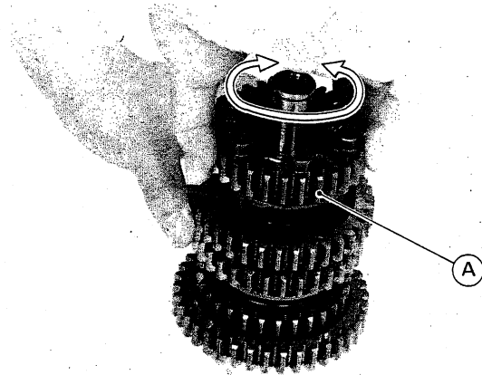
A. Zahnrad für den 5. Gang
