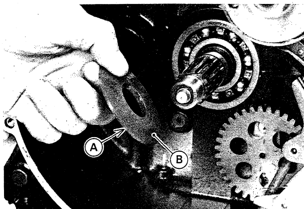
A. Distanzscheibe
