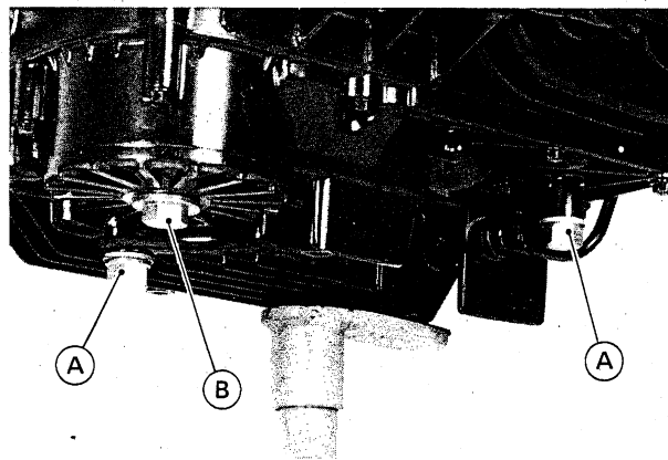
A. Ablasschraube B. Ölfilter-Befestigungsschraube
