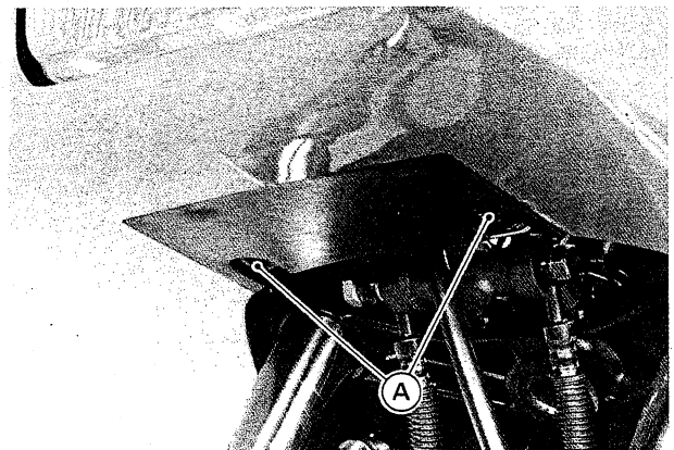
A. Schrauben für Abdeckung
