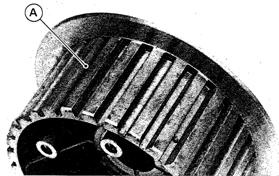
A. Keilverzahnung der Kupplungsnahe
