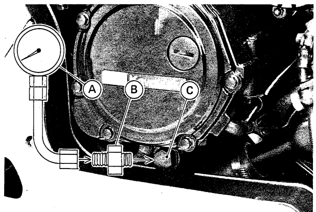
A. Öldruckmeßgerät: 57001-164
