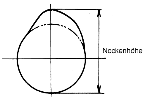
Messen der Nockenhöhe
