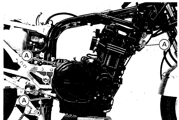
A. Befestigungsschrauben
