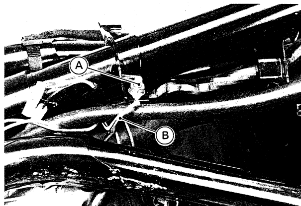
A. Geeignete Schraube oder Mutter B. Hauptkabelbaum-Masseleitung
