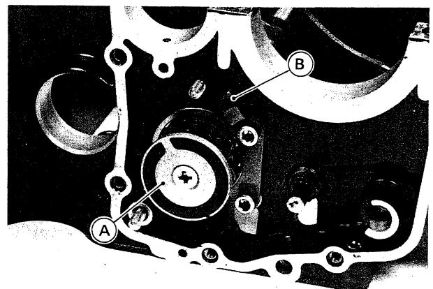
A. Schaltwalze
