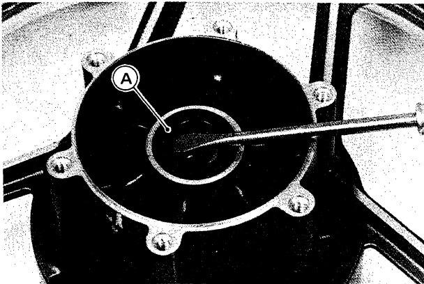
A. Fettdichtung
