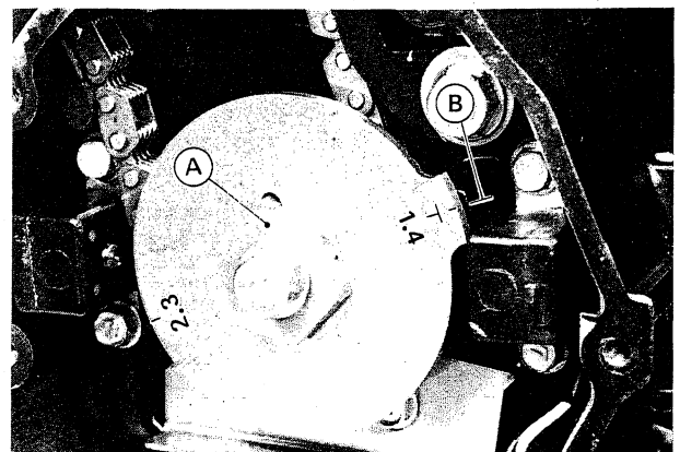
A. Mutter
