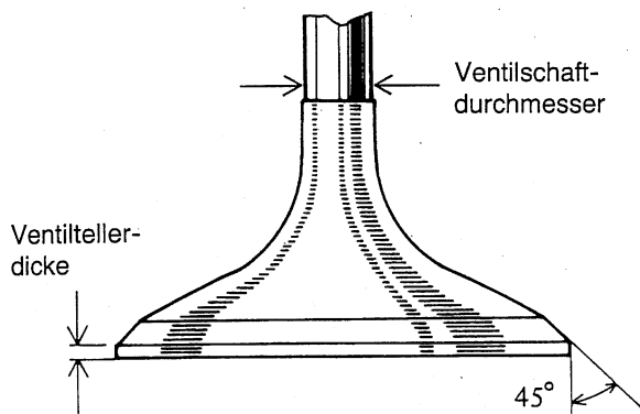
Ventilteller
