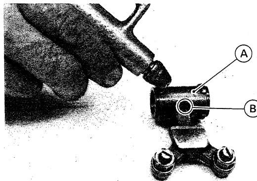
A. Schlepphebel
