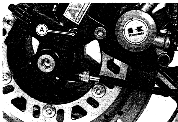
A. Ablassschraube
