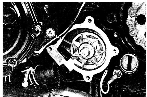
A. Flügelrad
