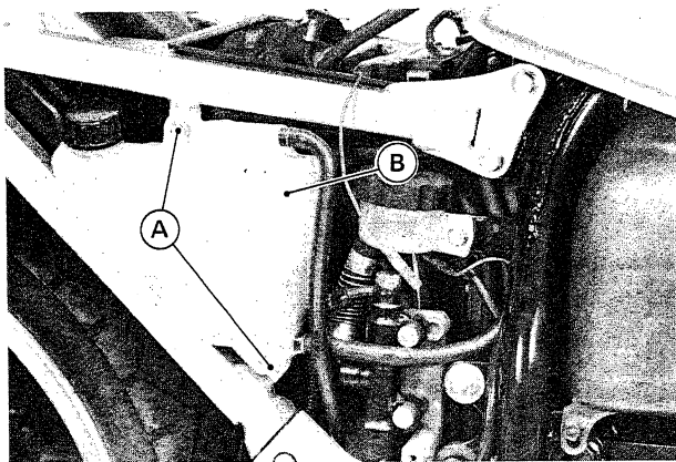
A. Schraube B. Reservetank
