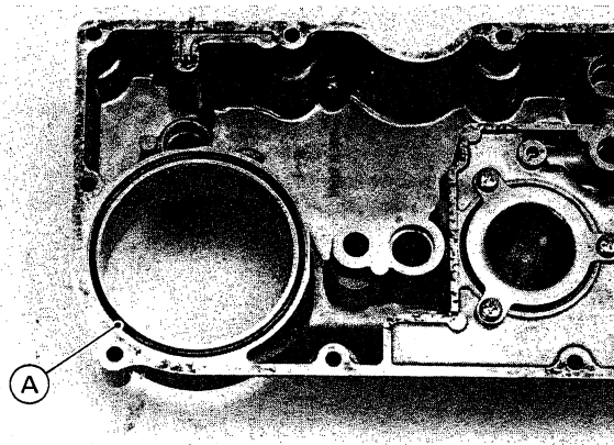
A. O-Ring
