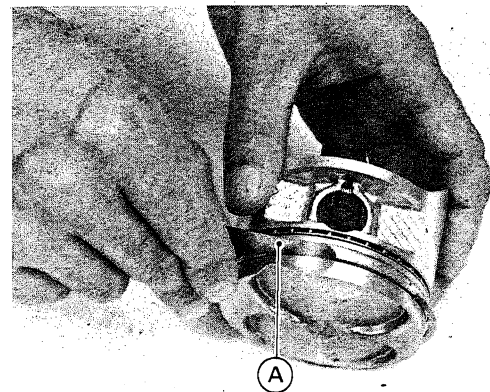
A. Fühlerblattlehre
