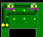
TX2720T CH PCB VER 2.0
